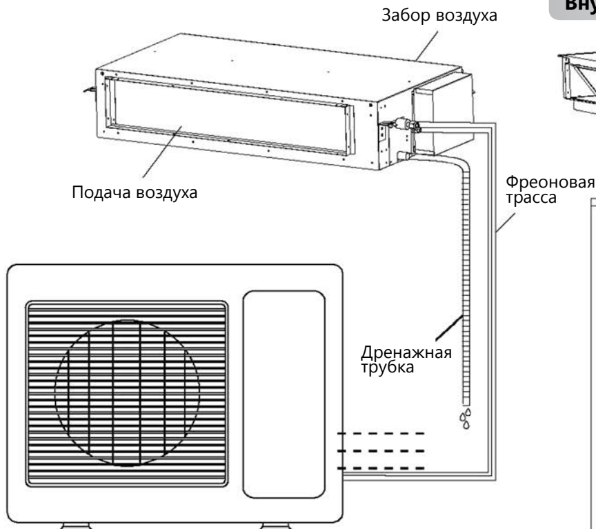
Внутренний блок (типоразмер 18/24/36)
