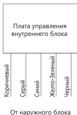
Клеммный терминал внутреннего блока
