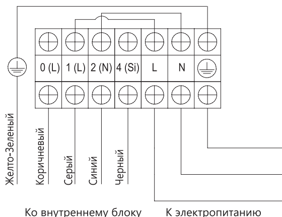
Клеммный терминал наружного блока
